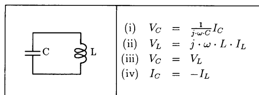
Fig. 8 Tuning circuit.
